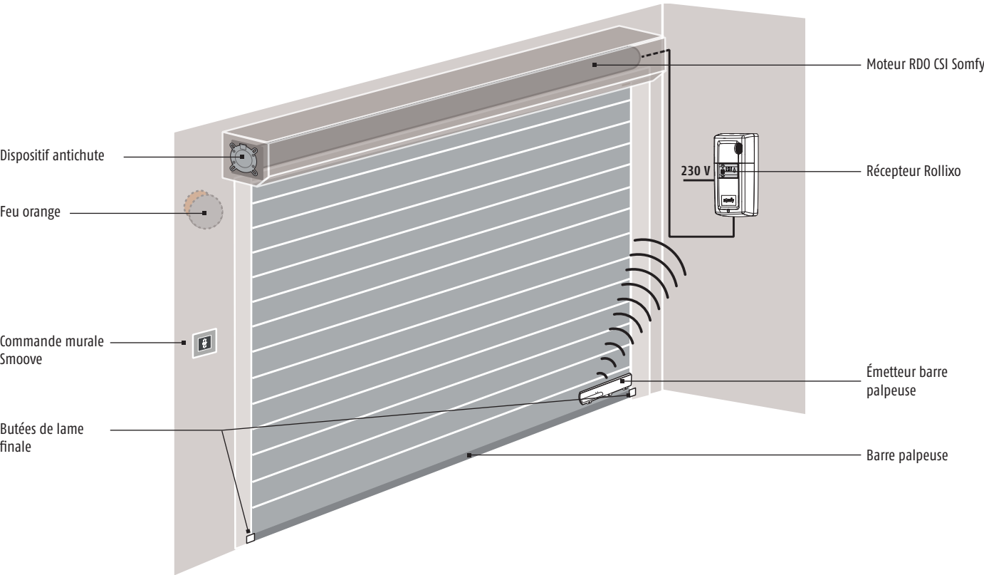
Schéma d'une installation Rollixo avec émetteur barre palpeuse optique
